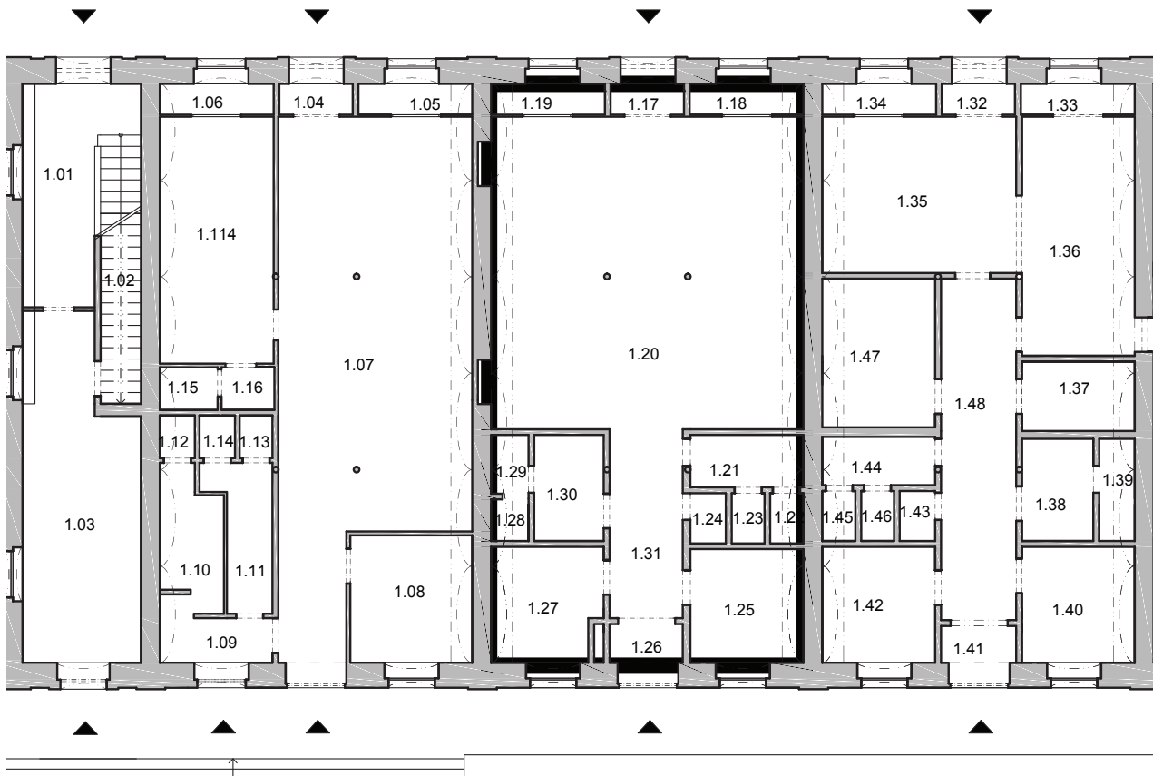
Schematický půdorys H18 1.NP
