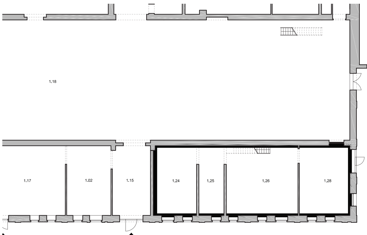
Schematický půdorys H13 1.NP
